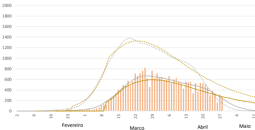
Figura 3. Análises para o dia 28 de abril utilizando os dois modelos, o inicial, que baseia as projeções nos últimos 14 dias, e o global que utiliza a informação de toda a série temporal através da equação descrita.
