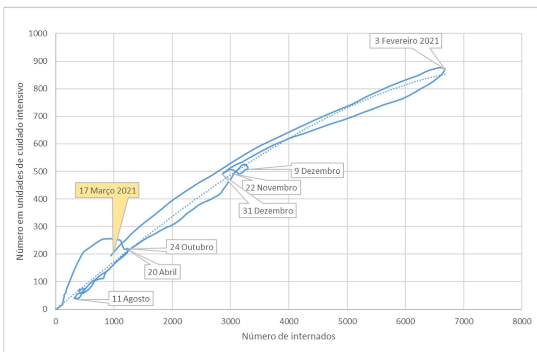
Figura 3. Relação entre a média semanal do número de internamentos e internamentos em cuidados intensivos três dias depois desde 1 de janeiro de 2020.
