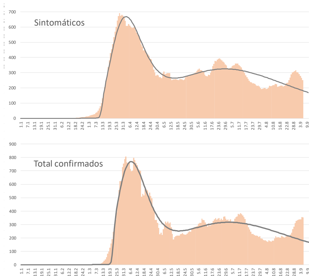
Figura 1. Evolução do número de casos sintomáticos e casos totais confirmados no País, mostrando o ajustamento dos modelos e indicando uma descida bastante clara, apesar dos números dos últimos dias que não contrariam ainda a tendência geral.
