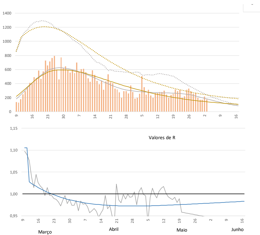
Figura 1. Análises para o dia 4 de junho utilizando os dois modelos, o inicial, que baseia as projeções nos últimos 14 dias, e o global que utiliza a informação de toda a série temporal através da equação descrita. O modelo global foi ajustado com os seguintes parâmetros e resultado:
