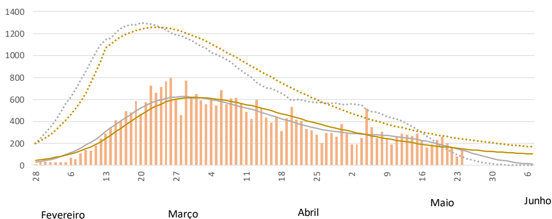
Figura 1. Análises para o dia 25 de maio utilizando os dois modelos, o inicial, que baseia as projeções nos últimos 14 dias, e o global que utiliza a informação de toda a série temporal através da equação descrita.
