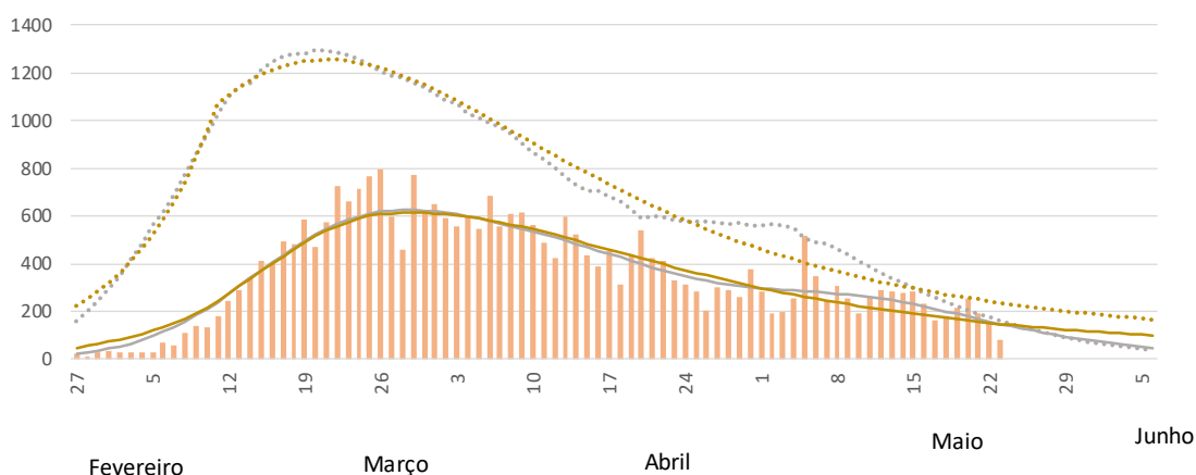
Figura 1. Análises para o dia 24 de maio utilizando os dois modelos, o inicial, que baseia as projeções nos últimos 14 dias, e o global que utiliza a informação de toda a série temporal através da equação descrita.
