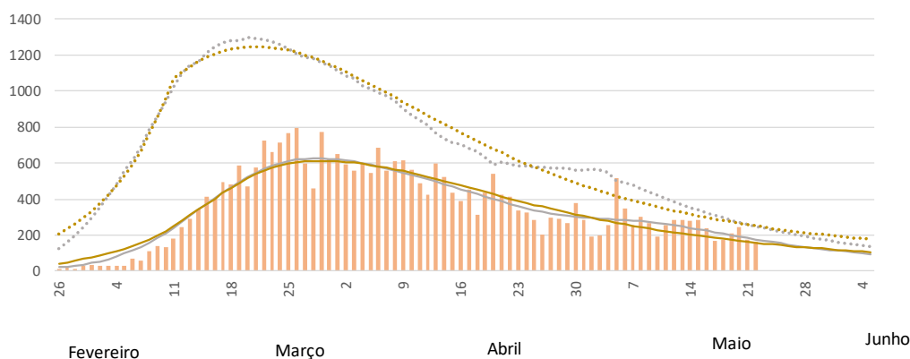
Figura 1. Análises para o dia 23 de maio utilizando os dois modelos, o inicial, que baseia as projeções nos últimos 14 dias, e o global que utiliza a informação de toda a série temporal através da equação descrita.
