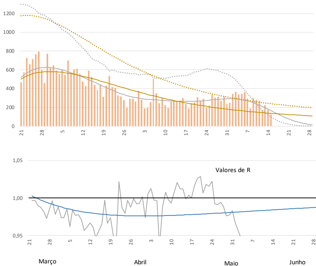
Figura 1. Análises para o dia 16 de junho utilizando os dois modelos, o inicial, que baseia as projeções nos últimos 14 dias, e o global que utiliza a informação de toda a série temporal através da equação descrita.
