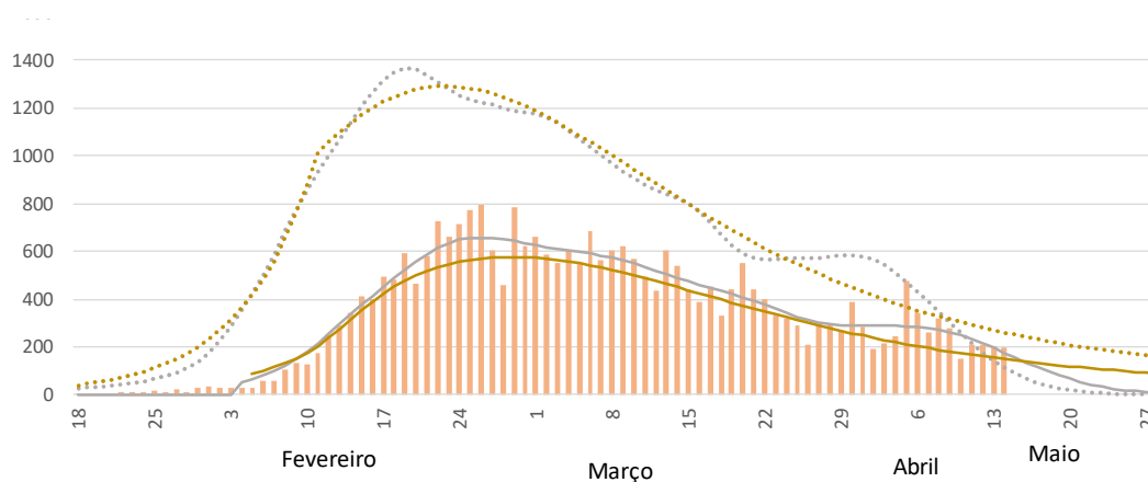
Figura 1. Análises para o dia 15 de maio utilizando os dois modelos, o inicial, que baseia as projeções nos últimos 14 dias, e o global que utiliza a informação de toda a série temporal através da equação descrita.
