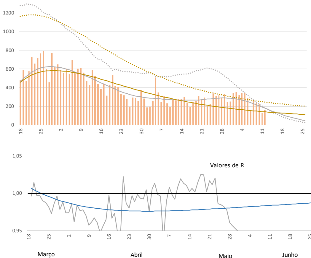
Figura 1. Análises para o dia 13 de junho utilizando os dois modelos, o inicial, que baseia as projeções nos últimos 14 dias, e o global que utiliza a informação de toda a série temporal através da equação descrita.
