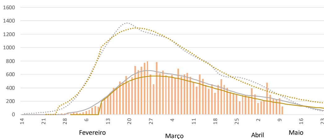
Figura 1. Análises para o dia 11 de maio utilizando os dois modelos, o inicial, que baseia as projeções nos últimos 14 dias, e o global que utiliza a informação de toda a série temporal através da equação descrita.
